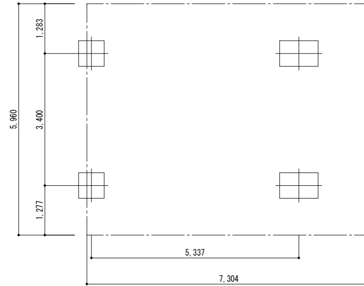
■ 基礎配置図
